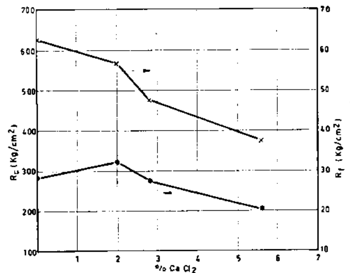
6 - Effetto della percentuale di \text{CaCl}_2 sulla resistenza meccanica a compressione ( R_c ) ed a flessione ( R_f ) del cemento pozzolanico.
